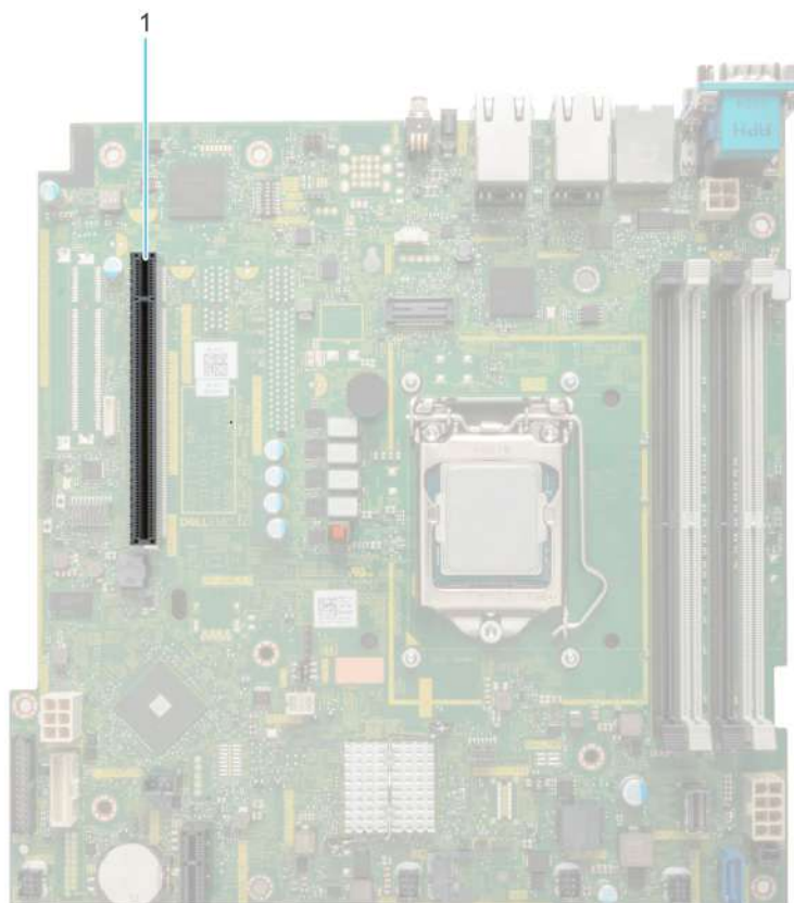
Ilustración 48. Conectores de la ranura de tarjetas de expansión
