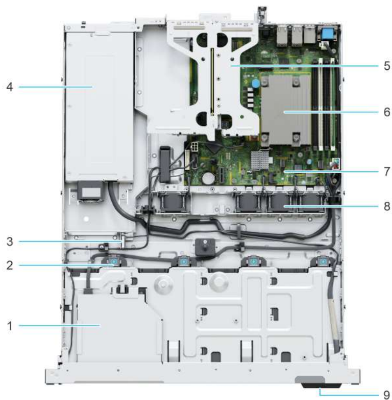
Ilustración 6. Vista interior del sistema de unidades cableadas
