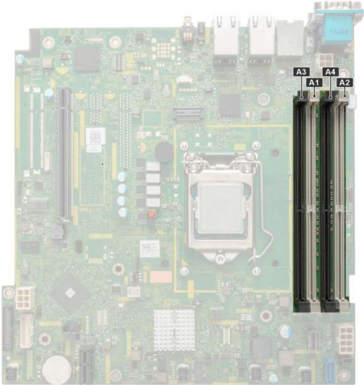
Ilustración 40. Ubicación de los conectores de memoria
