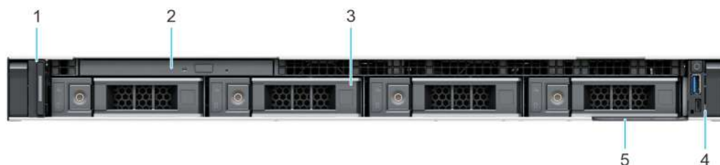
Ilustración 3. Vista frontal del sistema de 2 unidades SAS/SATA de 3,5 pulgadas cableado
