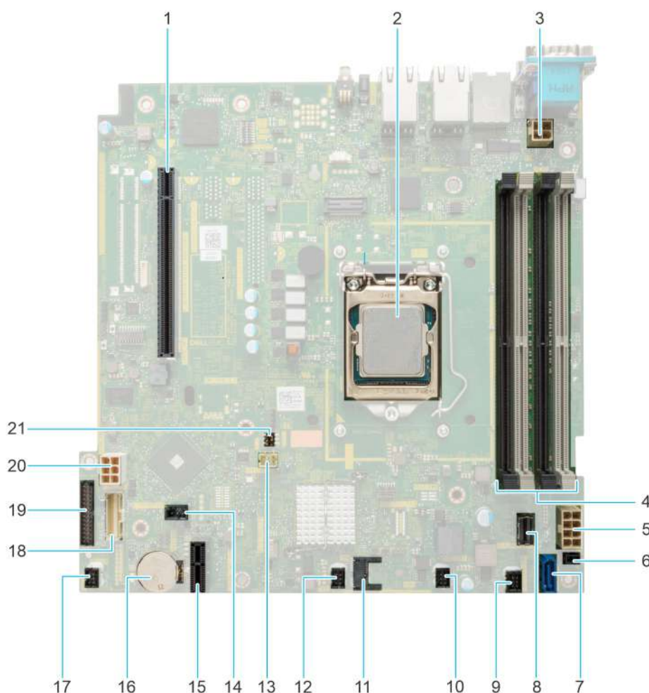
Ilustración 78. Puentes y conectores de la tarjeta madre
