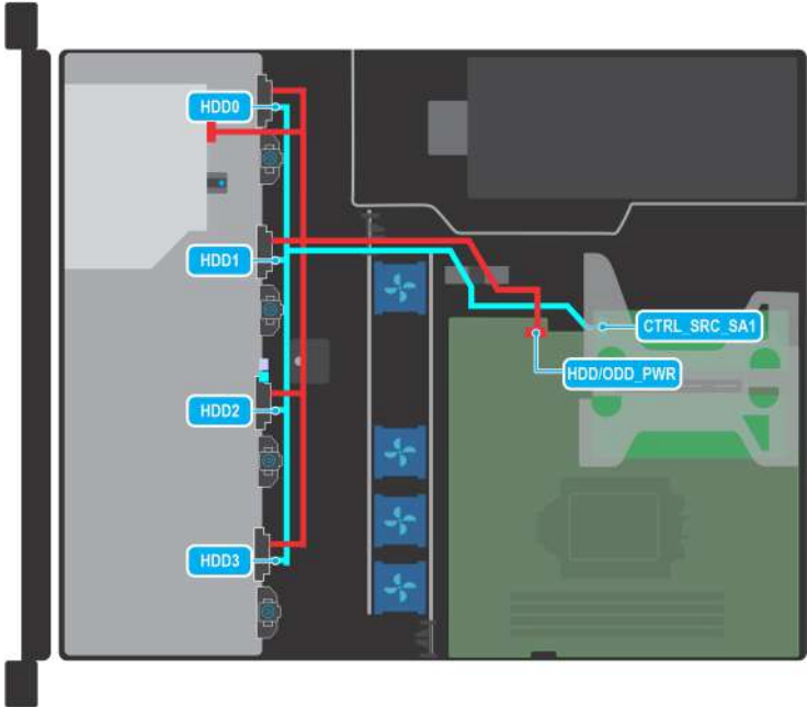
Ilustración 37. Colocación de los cables: configuración de la unidad cableada de 4 x 3.5 pulgadas con PERC
